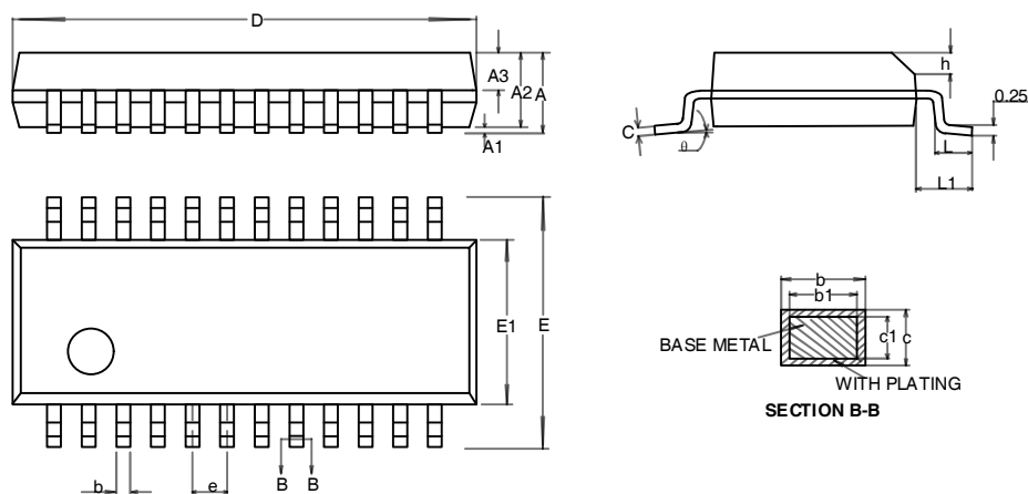
SSOP24 封装
