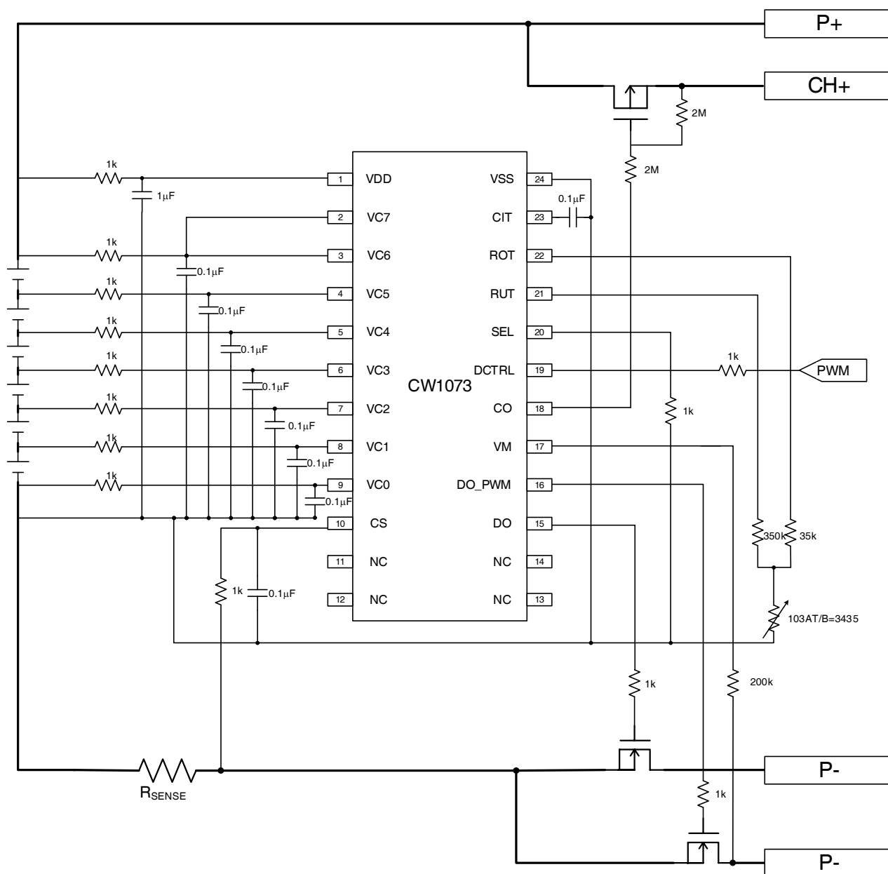
6 串不带均衡功能应用电路
