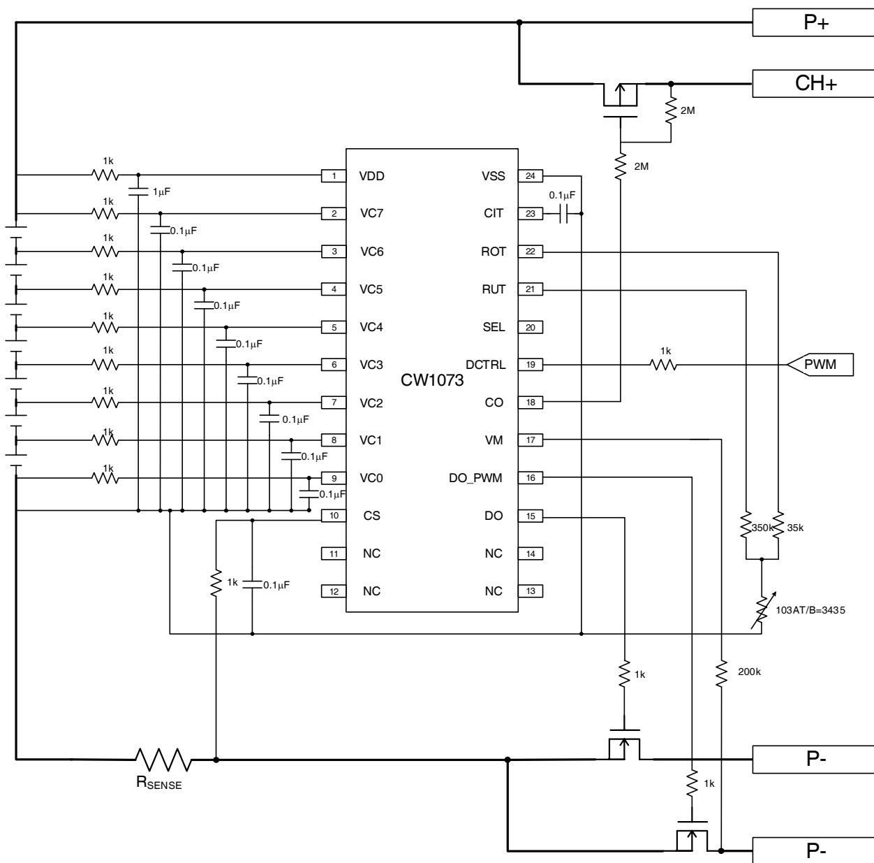
7 串不带均衡功能应用电路
